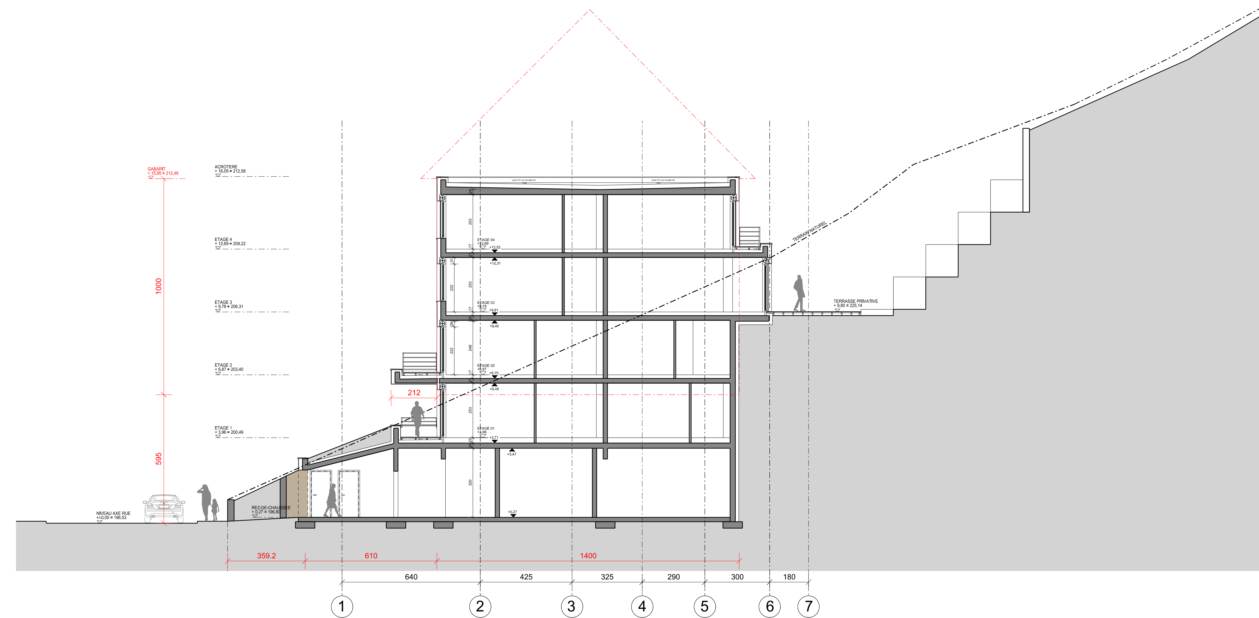
COUPE C-C
