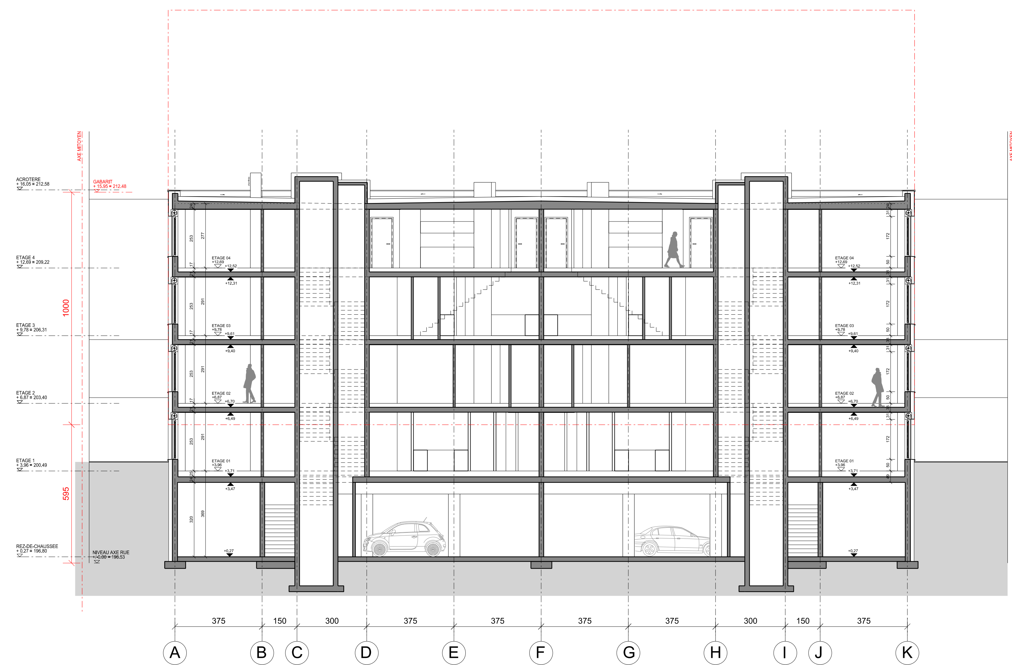
COUPE 1-1
