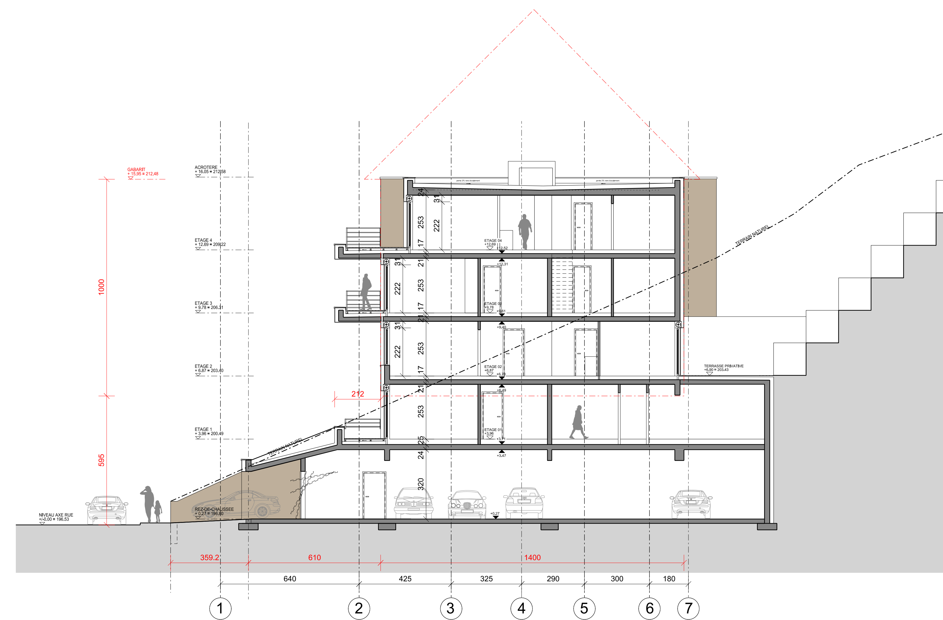
COUPE B-B
