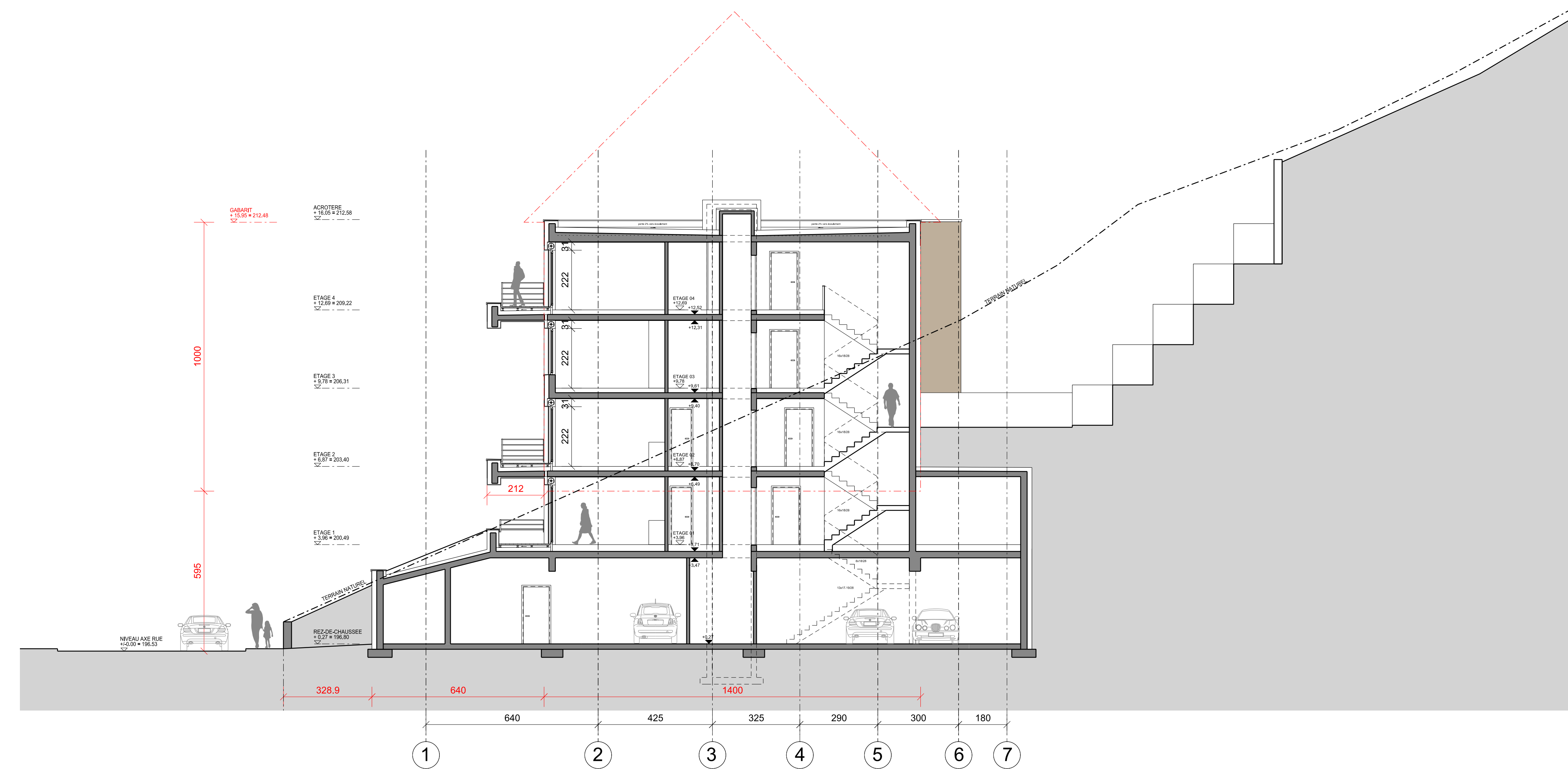
COUPE A-A
